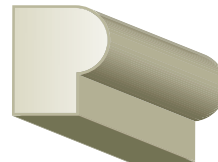
BA-409 ancho: 11.25cm (superior); 7.50cm (inferior) alto: 12.50cm
